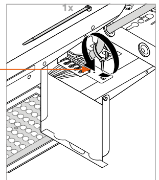
Grampo pré-montado para alívio de tensão do cabo de alimentação através de um simples grampo de cabo (não incluído)
