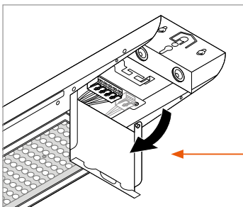
Abertura e fecho dos topos sem ferramentas que dão acesso a conectores elétricos
